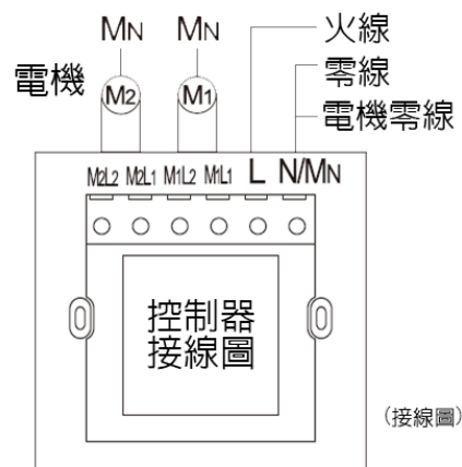
圖2 雙軌窗簾開關接線圖
